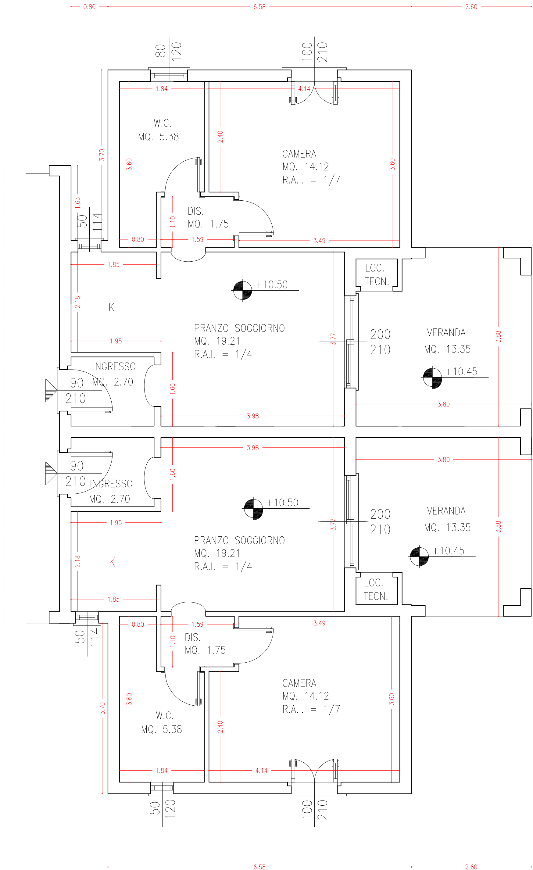
PIANTA PIANO TERRA – STATO DI FATTO
